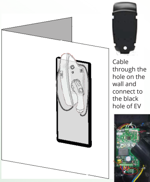
Wiring terminals
